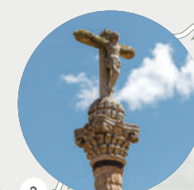
3 Cruz de Outeiro Outeiro
