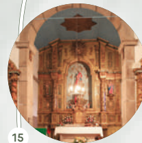
Igreja de São Pedro Avelanoso
