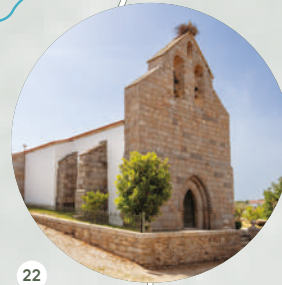
Igreja de Nossa Sra da Expectação Malhadas
