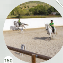
150 Centro Hecuestre Grijó
