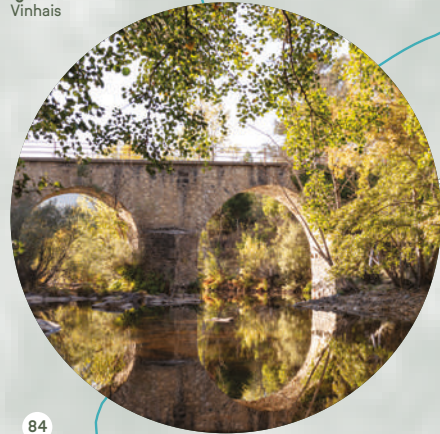
84 Ponte de Ranca Nunes
