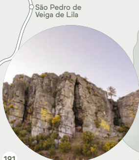
191 Buraco da Pala Passos
