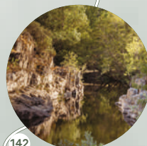
Pozo dos Paus Chacim
