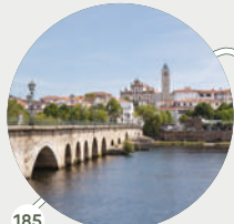
Puente Sobre o Tua Mirandela
