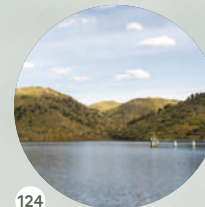
124 Presa de Santa Justa Eucisia
