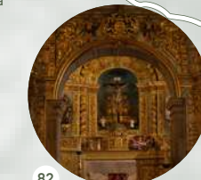
82 Igreja de São Pedro Zoio
