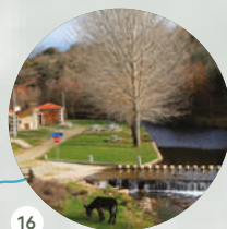
Zona de Ocio del Rio Angueira Angueira
