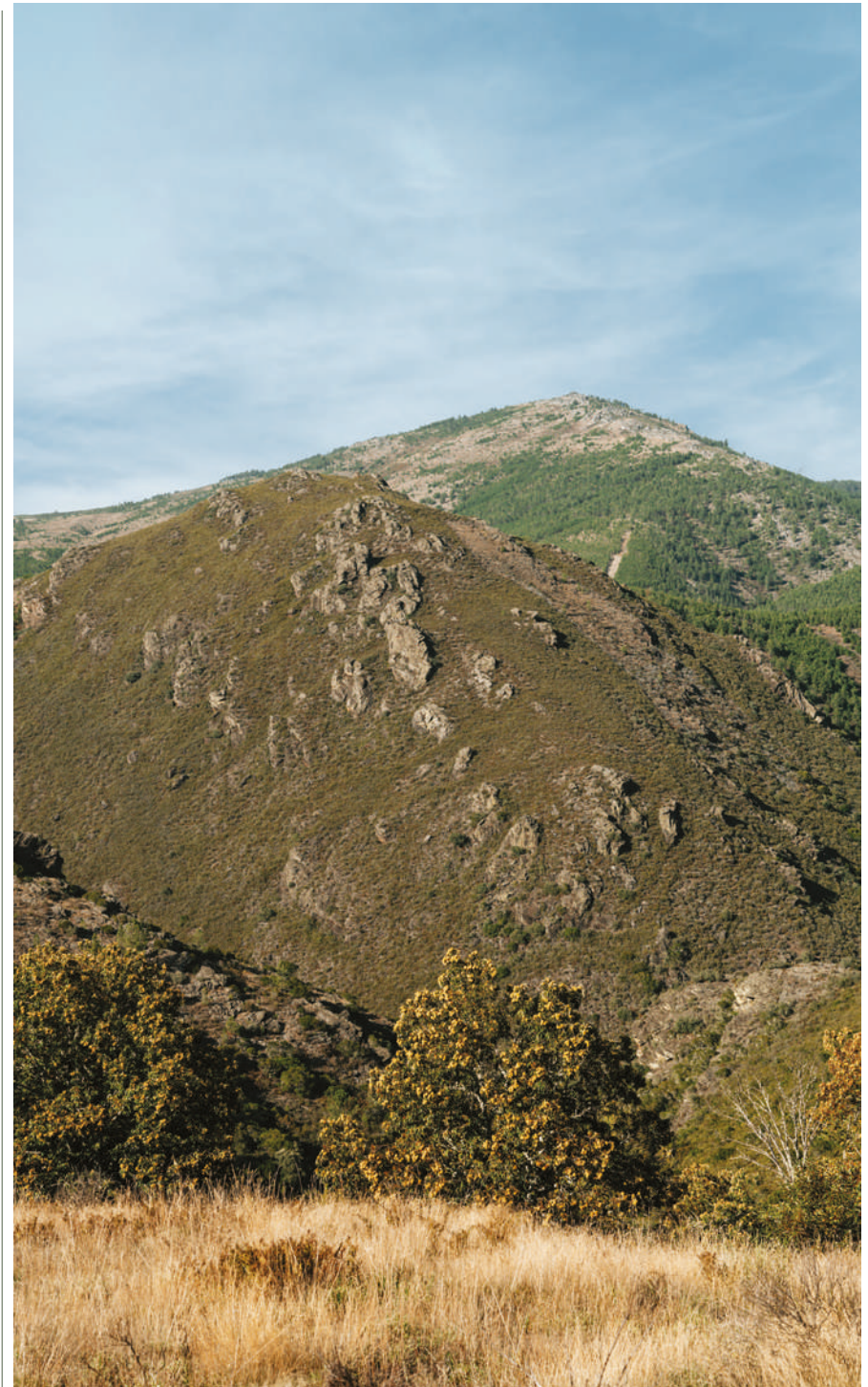
Ruta de la Terra Fria Transmontana
