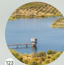
123 Presa de Salgueiro Vilarelhos
