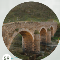
59 Puente Medieval Algo
