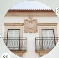
90 Museu de Arte Sacro Vinhais
