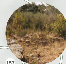
157 Terronha de Pinhovelo Pinhovelo El conjunto total de estructuras excavadas durante esta intervención arqueológica de emergencia sitúa la localidad de Terronha "como una de las estaciones romanas más imponentes del noreste de Portugal".
