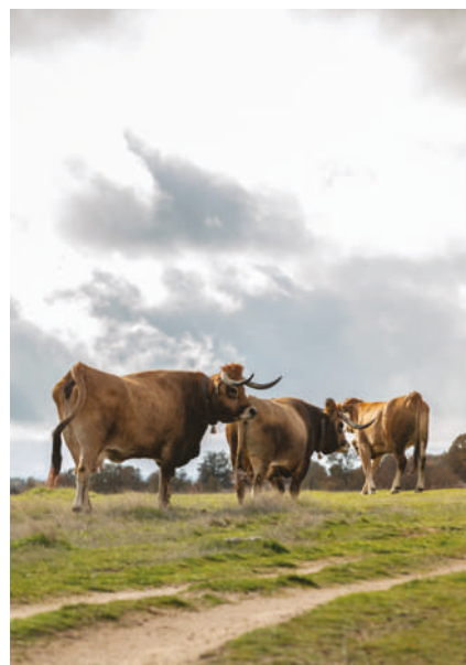
Raza bovina Mirandesa
