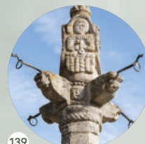
Picota de Chacim Chacim
